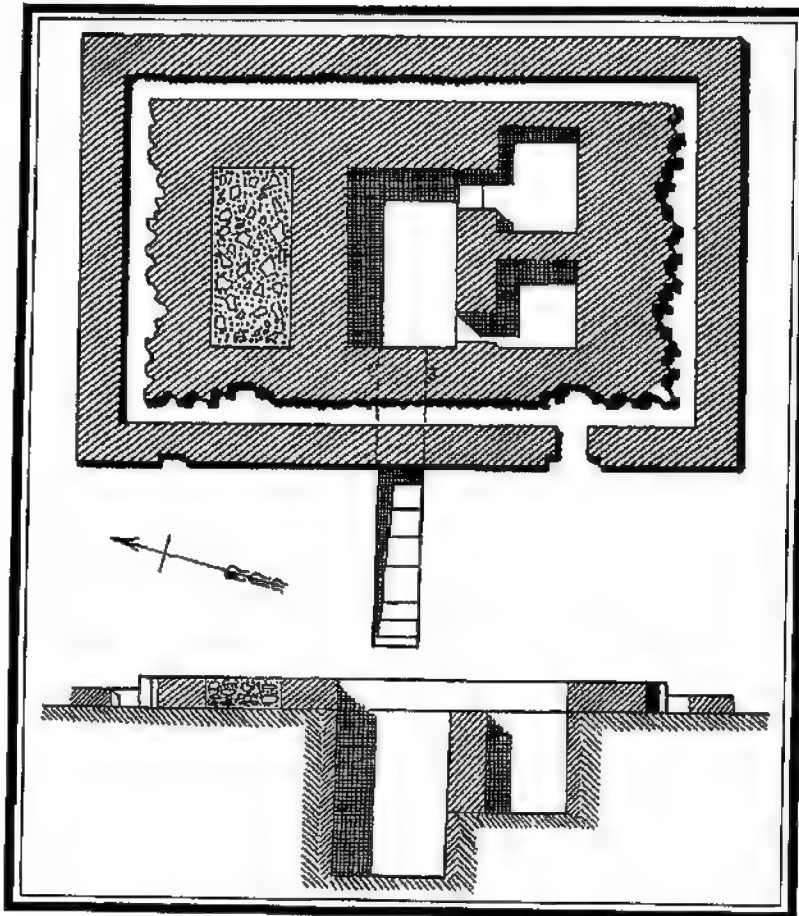
(شكل ٨٦) مسقطان أفقى ورأسى للمقبرة ١٣٧٤ في حلوان.
